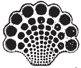
GRUSON. 10.717: en 1/2 plein G avec 1/2 boules
